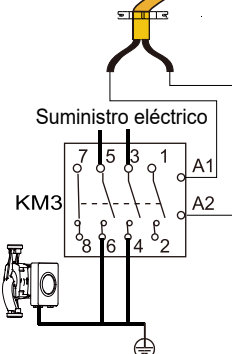
Bomba de circulación exterior P_o
