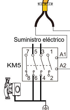
Bomba de tubería de ACS P_d
