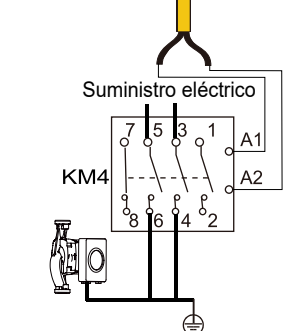
Bomba de energía solar exterior P_s.
